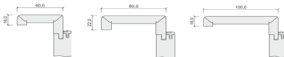
FU-RF 60/16 mm
