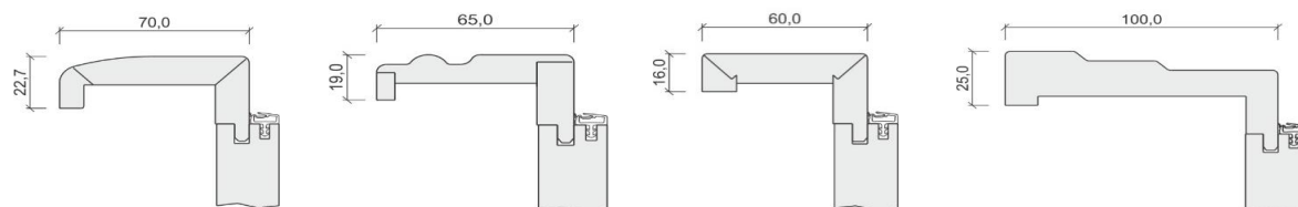
FU-SLF 70/22,7 mm
