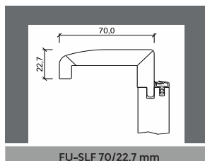
FU-SLF 70/22,7 mm
