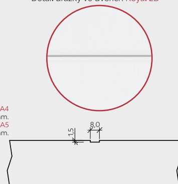
Detail drážky ve dveřích Royal 2D
