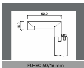
FU-EC 60/16 mm
