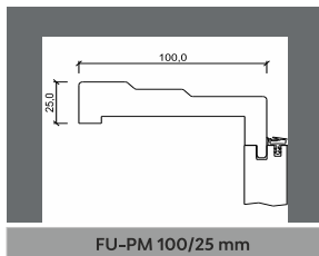
FU-PM 100/25 mm
