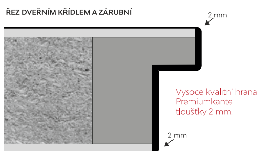
DVEŘNÍ KŘÍDLO S HRANOU PREMIUMKANTE (PK)
