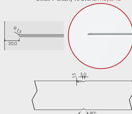
Detail V-drážky ve dveřích Royal 4D
