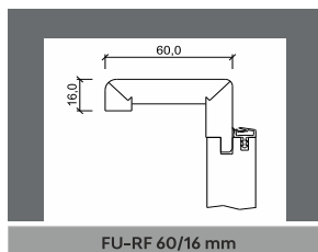
FU-RF 60/16 mm
