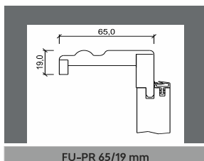
FU-PR 65/19 mm
