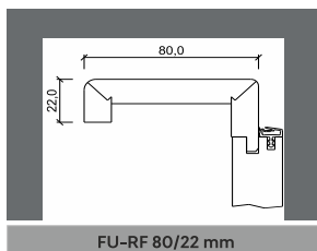
FU-RF 80/22 mm
