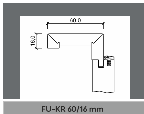
FU-KR 60/16 mm
