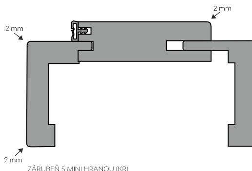
ZÁRUBEŇ S MINI HRANOU (KR)
