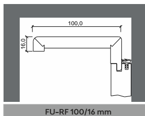
FU-RF 100/16 mm
