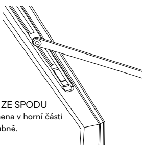
POHLED SHORA Detail Samozavírače zapuštěného do dveřního křídla.
