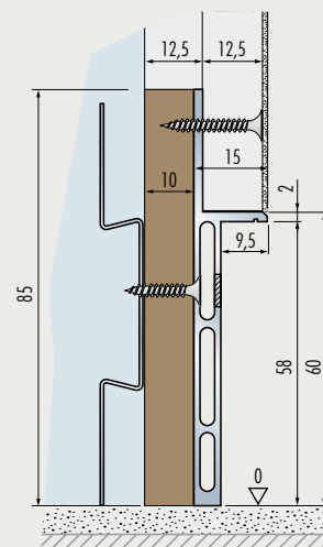
Soklový profil na SDK stěně při dvojitém opláštění
