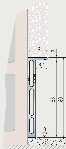
Soklový profil na zděné stěně
